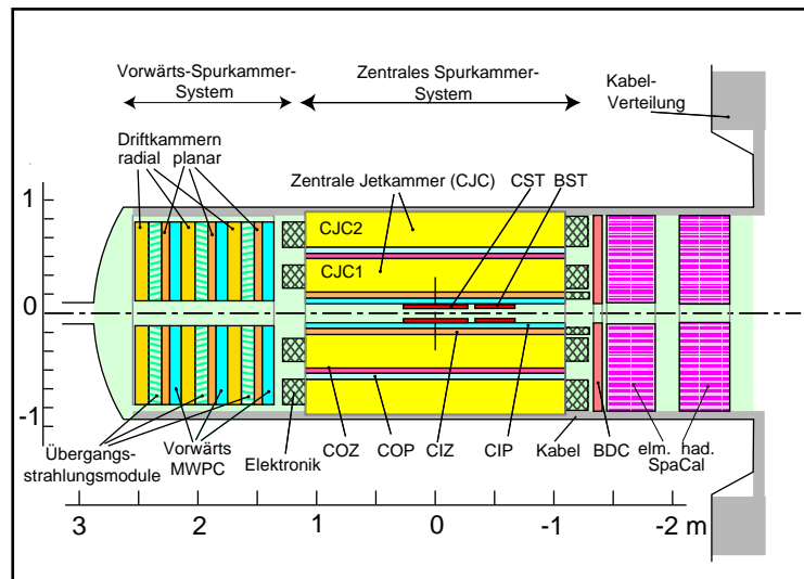
Abbildung 3.2: Das Spurdetektorsystem des H1-Detektors in Seitenansicht.
