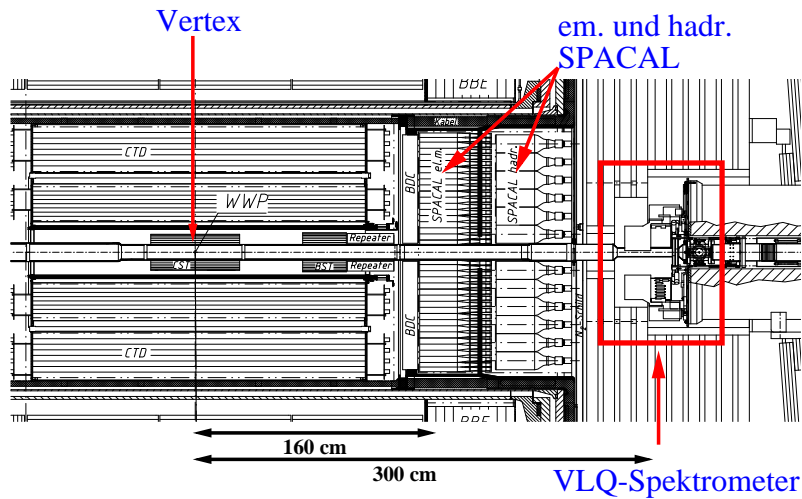
Abbildung 4.3: Maßstabgerechte Ansicht des VLQ-Spektrometers innerhalb des HI-Detektors. Der mit einem Quadrat markierte Bereich zeigt das VLQ-Spektrometer. Das Modul oberhalb des Strahlrohres ist in Meßposition und das untere Modul in der Position, in der es sich während der Injektionsphase befindet.
