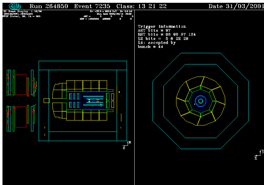
Abbildung 9.16: Gezeigt ist eines der verbleibenden Ereignisse in der H1-Ereignisdarstellung. Der H1-Detektor ist “leer”, daß heißt, keine Spuren in den Spurkammersystemen und keine Energiedeposition in den Kalorimetern, mit Ausnahme des SPACAL-Kalorimeter. Die Energiedeposition durch das \pi^0 -Zerfallsphoton im SPACAL-Kalorimeter ist in dieser Darstellung wegen seiner geringen Energie nicht zu erkennen. Aus der Variablen “AST” (actual-subtrigger) ist abzulesen, daß das Ereignis durch den Subtrigger zur Odderonsuche S97 akzeptiert wurde.
