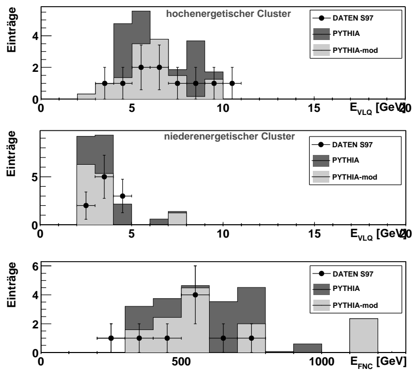
Abbildung 10.6: Es sind dieselben Kontrollverteilungen wie in Abbildung 10.5 gezeigt, diesmal für Ereignisse aus den TT , BB -Kanälen. Auch hier findet sich eine akzeptable Übereinstimmung zwischen Daten und Monte-Carlo.
