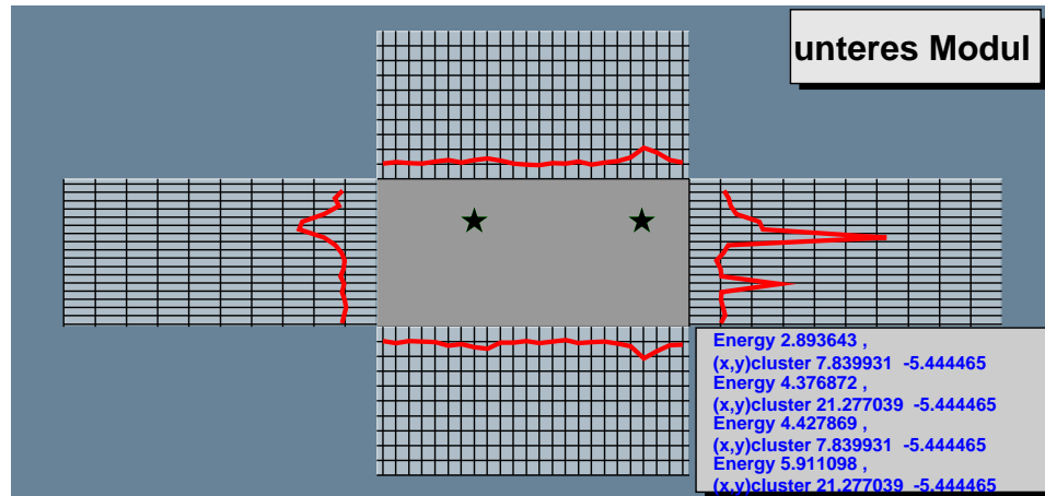
Abbildung 9.17: Darstellung des einzig verbleibenden Ereignisses im TT-Kanal in der VLQ-Kalorimeter Ereignisdarstellung. Die rekonstruierte \gamma\gamma -Masse betr\u00e4gt m_{\gamma\gamma} = 0.184 \text{ MeV}
