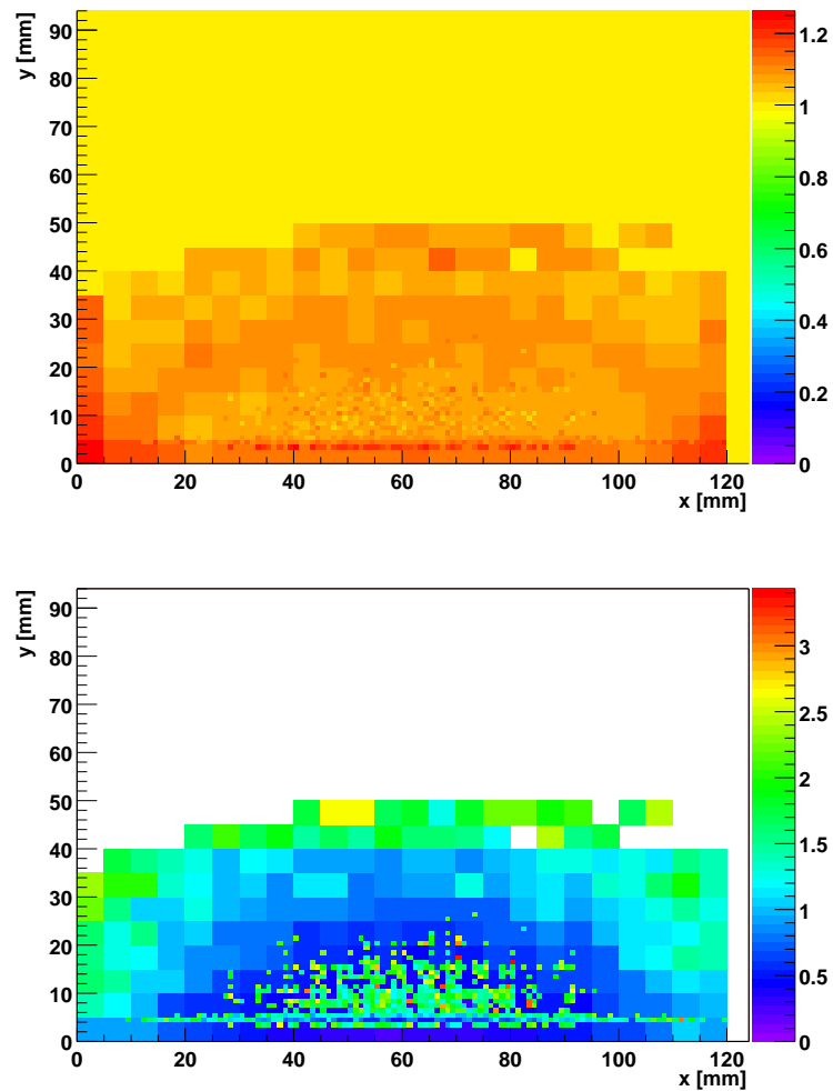
Abbildung 7.11: Gezeigt ist eine zu Abbildung 7.10 analoge Darstellung der absoluten Kalibrationsfaktoren und deren Fehler für Monte-Carlo simulierte Ereignisse aus dem kinematischen Maximum. Lauflängeneffekte im Szintillator werden in der Monte-Carlo Simulation zwar berücksichtigt, aber unterschätzt. Entgegen Kalibrationsfaktoren die aus den echten Daten nahe des Randes bestimmt wurden, sind hier deutlich größere Korrekturfaktoren am Rand ermittelt worden. Ganz besonders deutlich wird es an den Ecken, an denen der Schauer an zwei Flächen aus dem Kalorimeter austreten kann. Zum Inneren des Kalorimeters hin nähern sich die Kalibrationsfaktoren dem Wert 1.0. Der Grund liegt in der Eichung der Detektorantwort der Simulation auf die Elektronstrahlenergie im Zentralbereich des Kalorimeters.
