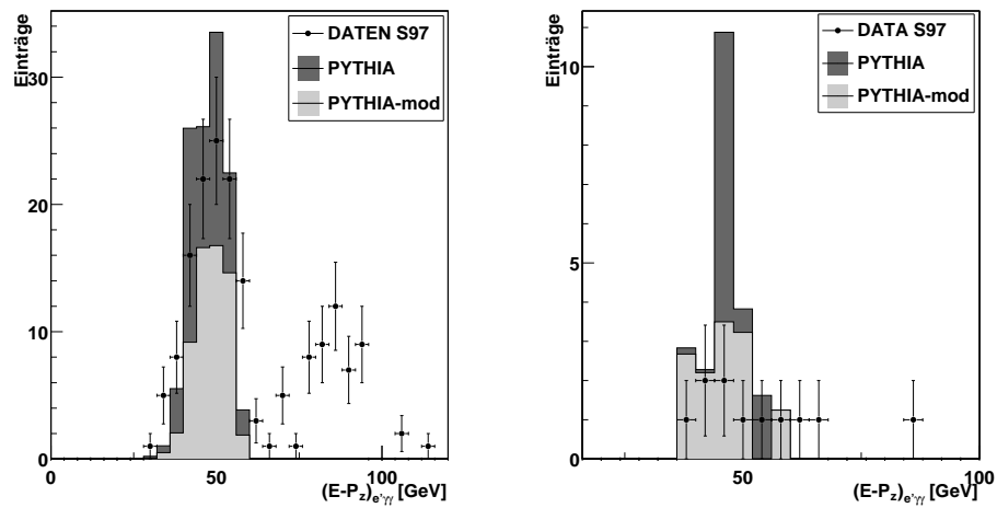
Abbildung 10.7: Die Verteilung in der Variablen in der E - p_z für gemessene und simulierte Ereignisse. Bedingt durch die in Kapitel 8.4 beschriebenen Schnitte in der Generation der Ereignisse, findet man nur Ereignisse mit einem Wert von E - p_z > 40 . Die Ereignisse bei E - p_z > 70 sind Doppelereignisse die nicht simuliert werden. Die durch das Monte-Carlo PYTHIA vorhergesagte Verteilung, ist in beiden Kanälen mit der tatsächlich beobachteten, verträglich.
