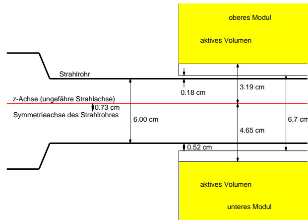
Abbildung 4.5: Resultierende Anordnung der VLQ-Kalorimetermodule und des HERA-Elektronstrahles nach der Ortskalibration mit QED-Compton Ereignissen. Das untere Modul befindet sich generell weiter vom Strahl entfernt als das obere Modul. Zu den Abständen müssen die Positionsangaben der Fahrmechanik addiert werden.
