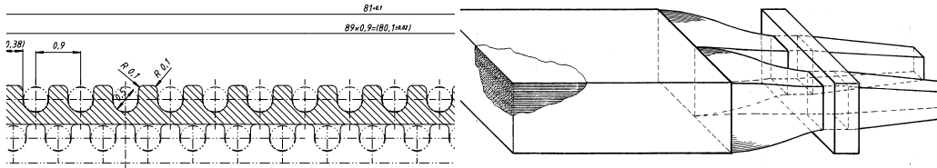
Abbildung 3.3: Im linken Bild ist eine Frontansicht auf die Blei-Faser Matrix des SPACAL zu sehen. Die Fasern fungieren als aktives Material. Das rechte Bild zeigt den Aufbau eines Submoduls. Das Licht aus den Fasern wird über Faserbündel zu einem Lichtmischer geleitet. Sie werden durch Photomultiplier ausgelesen.
