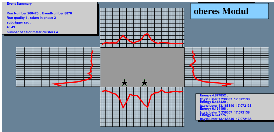
Abbildung 6.5: Ein Ereignis aus den echten Daten bei dem zwei Teilchen in einer Ebene parallel zur horizontalen Projektion aufgetroffen sind. Entgegen zu dem in Abbildung 6.4 gezeigten Ereignis ist in diesem Fall eine eindeutige Ortsrekonstruktion möglich. Die Energie der beiden Cluster kann jedoch nicht eindeutig bestimmt werden, da beide Teilchen in den beiden vertikalen Projektion ihre Energie in denselben Kanälen hinterlassen. Die Rekonstruktion teilt die Energie in der vertikalen Projektion gemäß dem Verhältnis der Energien der beiden Cluster in den horizontalen auf.
