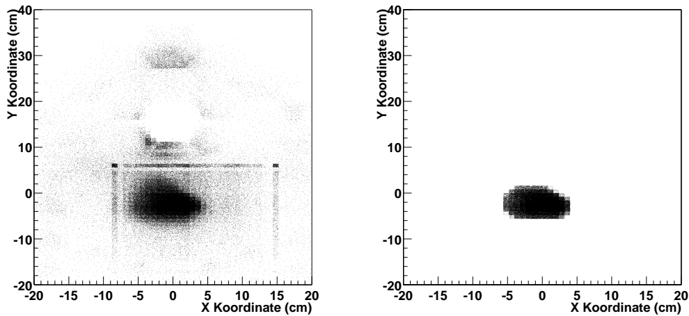
Abbildung 9.15: xy -Karte der Trefferverteilung auf dem FNC Kalorimeters vor und nach der Neutronselektion. Der Bereich um x = 0 cm und 10 cm < y < 20 cm, in dem keine Treffer zu sehen sind, ist die Protonstrahlröhre. Der Bereich erhöhter Trefferdichte oberhalb der Protonstrahlröhre stammt von Protonen, deren Energien von der nominellen Protonenergie so stark abweicht, daß sie vor dem FNC-Kalorimeter nicht mehr ausreichend abgelenkt werden können. Die Schnitte selektieren Ereignisse, die in einer Region des FNC-Kalorimeters liegen, deren Akzeptanz für Neutronen größer als 90% ist.
