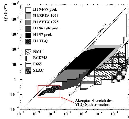
Abbildung 4.2: Die kinematische Akzeptanz des HI-Detektors in der (x_{Bj}, Q^2) -Ebene. Zum Vergleich sind noch die kinematischen Bereiche einiger Fixed-Target-Experimente abgebildet. Der VLQ-Detektor erweitert den Meßbereich des HI-Detektors im Bereich kleiner Werte von Q^2 und x_{Bj} .
