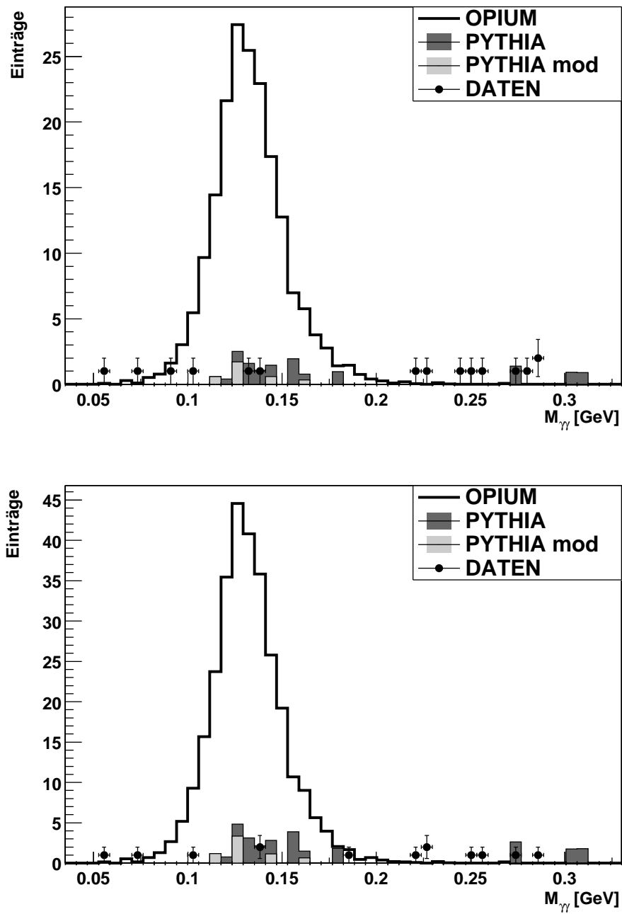
Abbildung 10.3: Das \gamma\gamma -Massenspektrum der Daten nach Kombination der Kanäle TT, BB, VS und akzeptiert durch die Subtriggern S96 (oberes Bild) und S97 (unteres Bild). Die erwarteten und gemessenen Ereigniszahlen sind in Tabelle 10.1 angegeben.
