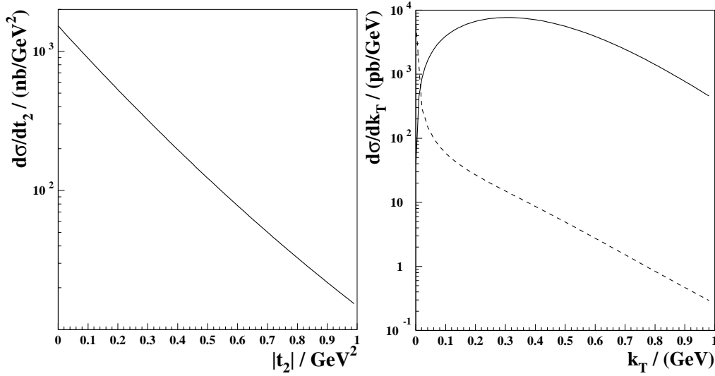
Abbildung 1.15: Links: Vorhergesagter Wirkungsquerschnitt d\sigma_{\gamma p}^{\omega}/dt für den Prozeß \gamma p \rightarrow \pi^0 N^* als Funktion von t .
