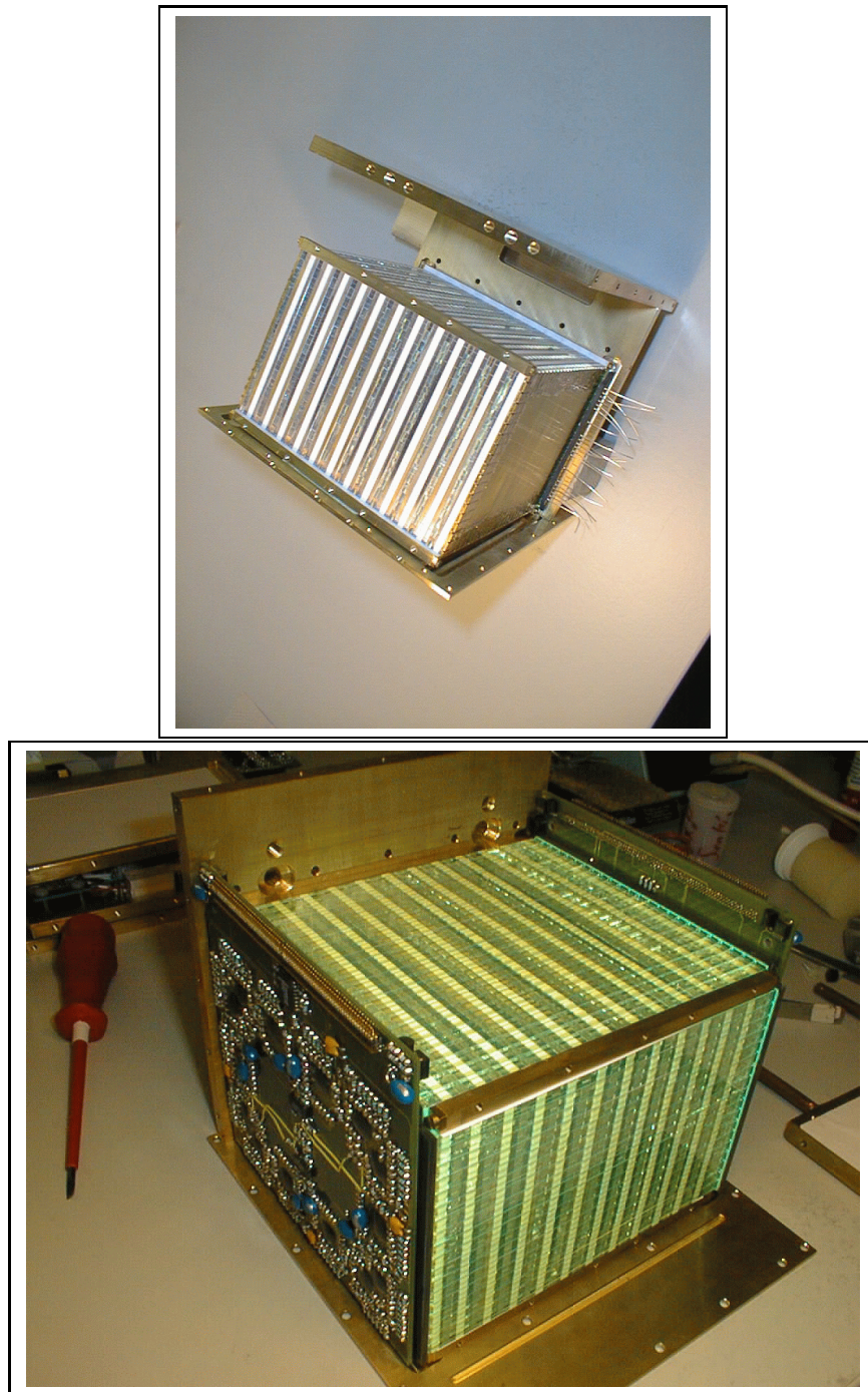
Abbildung 5.2: Die obere Photographie zeigt die aktive Struktur eines VLQ-Kalorimeters Moduls. Die abwechselnden Lagen von Szintillatorstäben und Wolfram Platten sind deutlich zu erkennen. Die “weißen” Schichten sind in Papier eingewickelten Szintillatoren. Die abwechselnde Orientierung der Szintillatorlagen ist aus den abwechselnd weißen und “durchsichtigen” Schichten ersichtlich. Die untere Photographie zeigt ein fast vollständig zusammengesetztes VLQ-Kalorimetermodul bei dem die Wellenlängenschieber und Photodiodenzeilen bereits montiert sind. Die Wellenlängenschieber sind so angeordnet, daß sie das Licht aus den Szintillatoren entlang der longitudinaler Schauerachse aufsummieren. Durch die Segmentierung wird das transversale Schauerprofil gemessen. Die Wellenlängenschieber sind durch zwei Führungsschienen fixiert. An den Stirnseiten sind zwei PCB-Platinen mit Teilen der Ausleseelektronik montiert.
